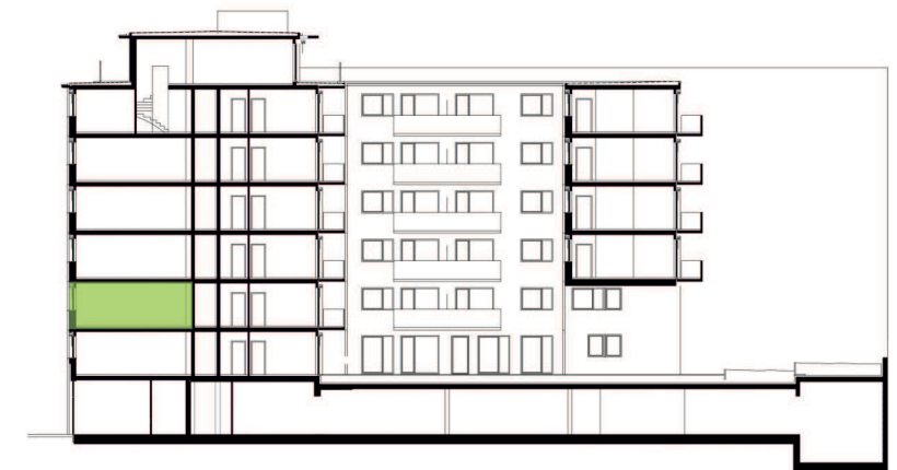
metszet
