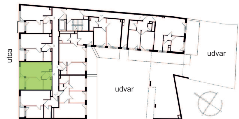
átnézeti alaprajz
